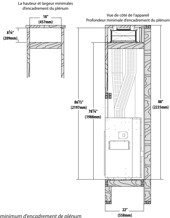
FIGURE 2.10 Dégagements et dimensions minimum d'encadrement de plénum pour le foyer BHM-38
