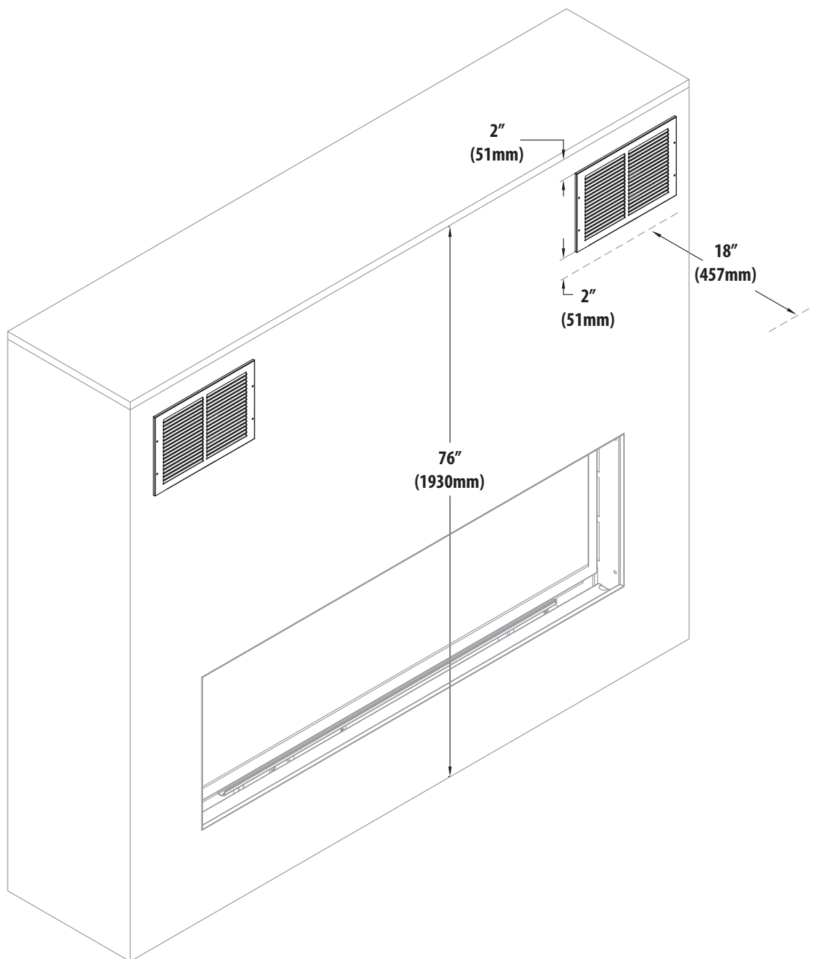
FIGURE 2.13 Dégagements aux mur face avant de CLW-ST
