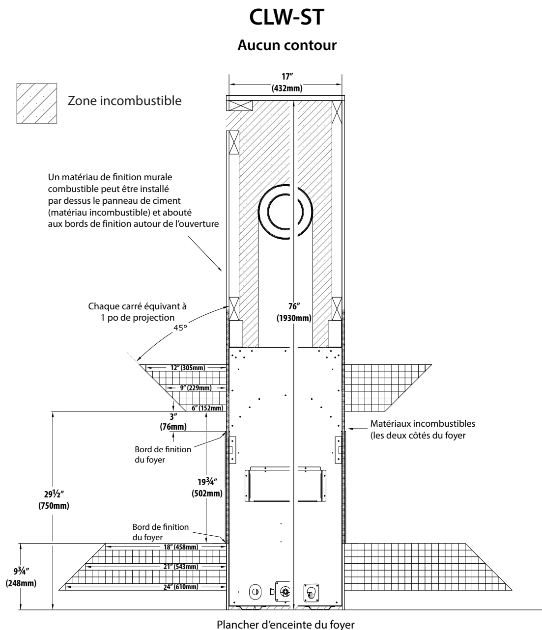
FIGURE 3.11 Dégagements de l'âtre et du manteau pour une installation sans contour pour le foyer CLW-ST
