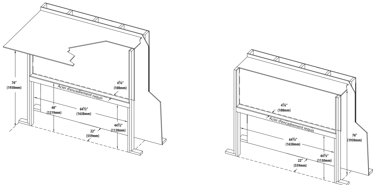
FIGURE 2.4 Encadrement et dégagement pour le foyer CLW-50
