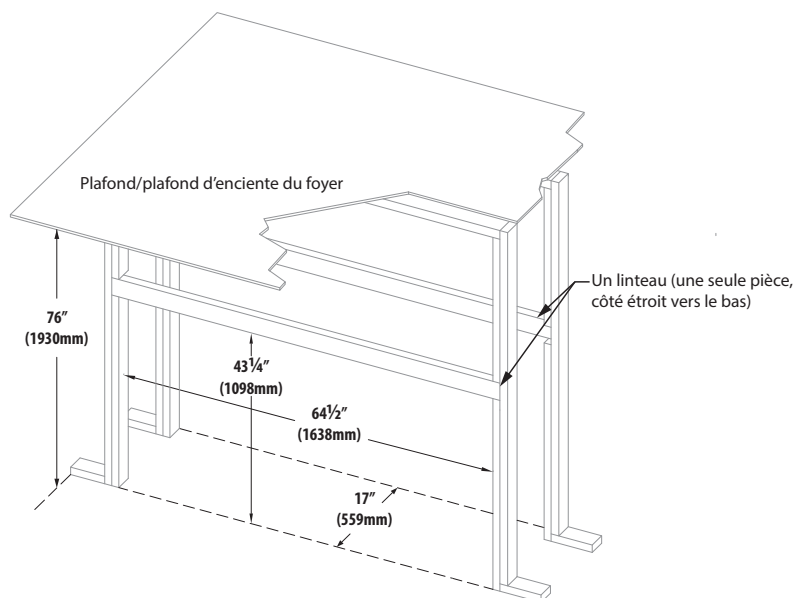
FIGURE 2.6 Encadrement et dégagement pour le foyer CLW-ST
