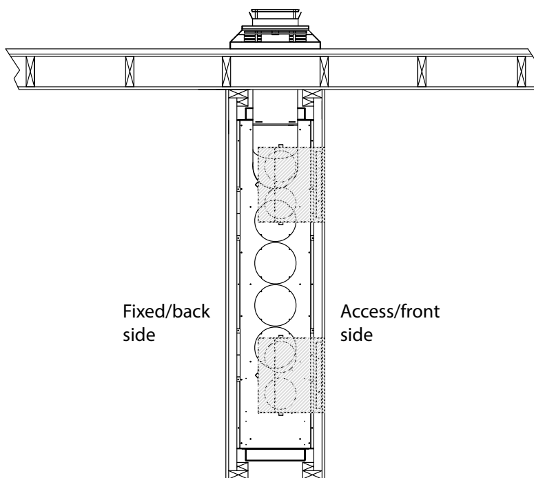
FIGURE 1.5 CLW-ST Configurations suggérées du KZK-1510A
