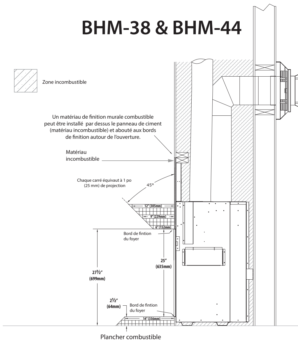
FIGURE 3.12 Dégagements de l'âtre et du manteau pour une installation sans contour pour le foyer BHM-38 et BHM-44
