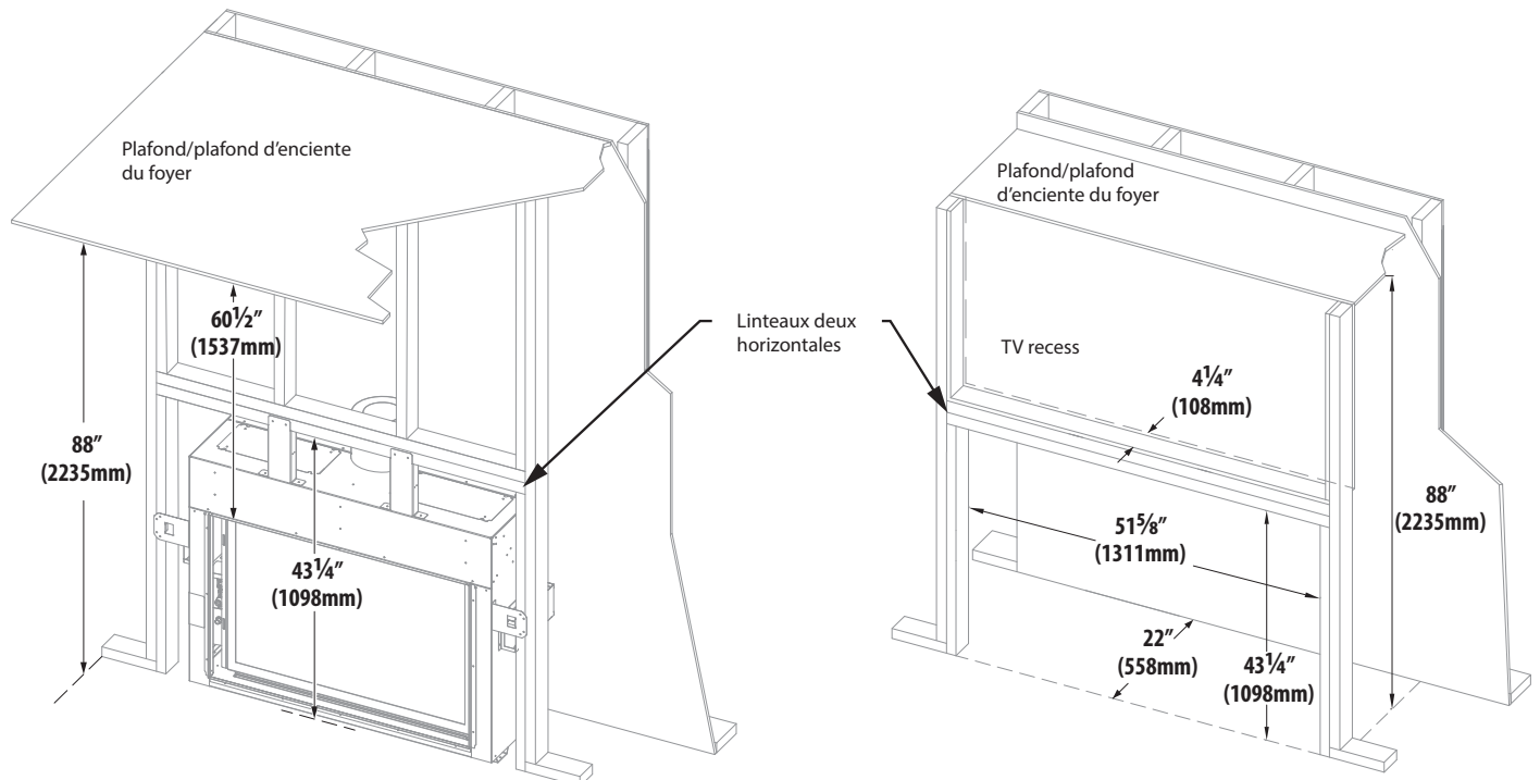
FIGURE 2.9 Encadrement et dégagement pour le foyer BHM-38
