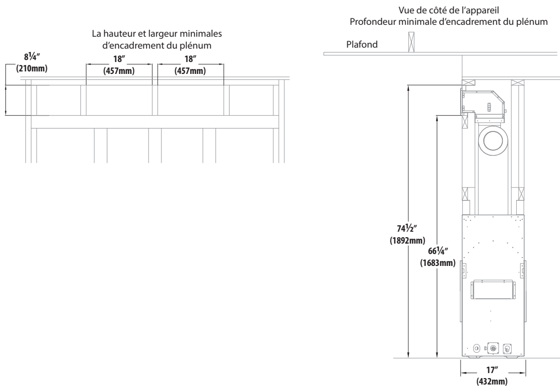
FIGURE 2.5 Dégagements et dimensions minimum d'encadrement de plénum pour le foyer CLW-ST
