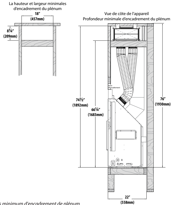
FIGURE 2.3 Dégagements et dimensions minimum d'encadrement de plénum pour le foyer CLW-50
