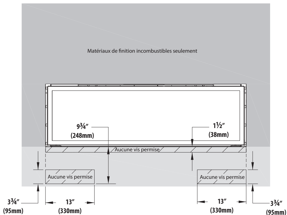
FIGURE 3.1 Dimensions minimales des matériaux incombustibles de finition pour le foyer CLW-50
