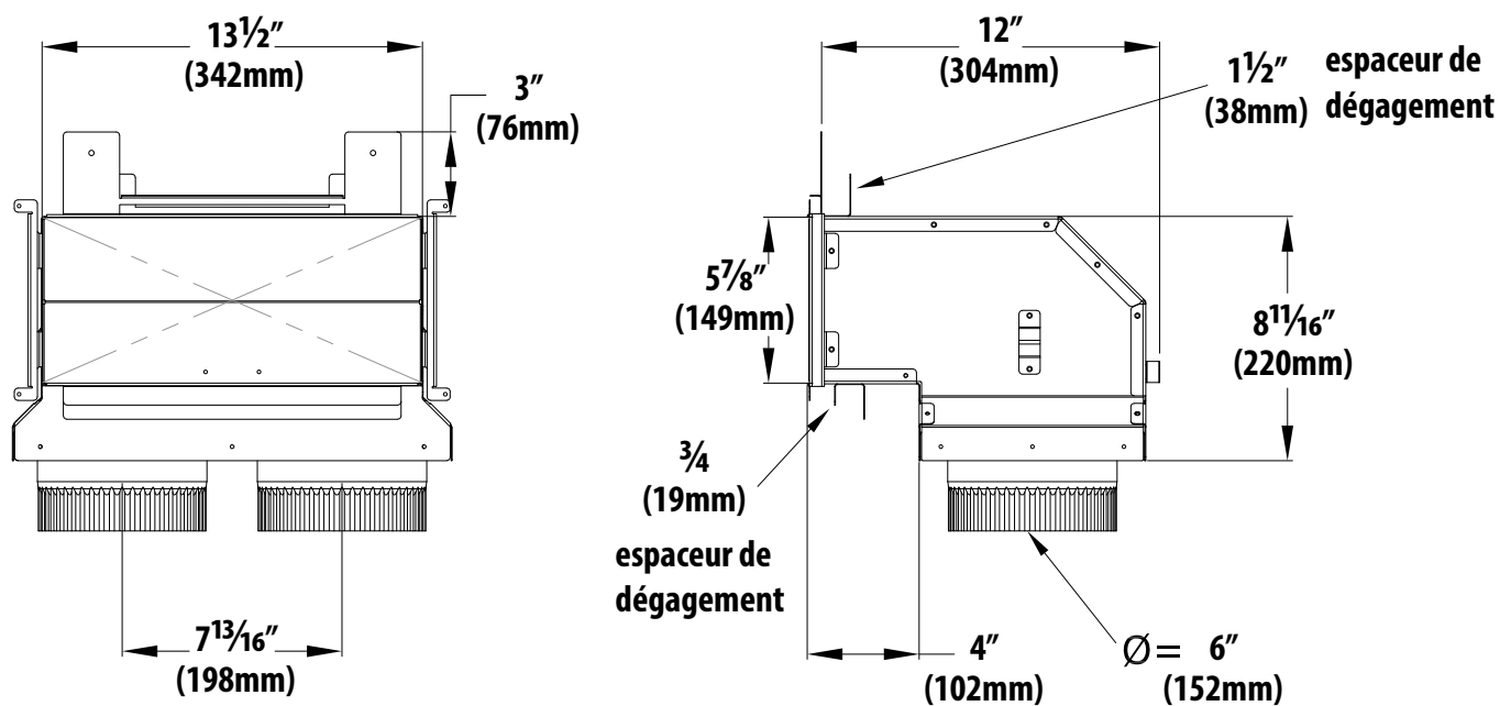
FIGURE 1.7 Dimensions du KZK-1510A
