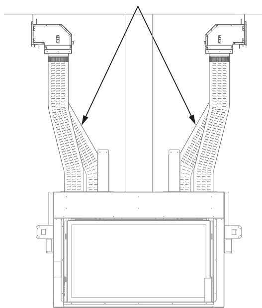
FIGURE 1.6 BHM-38 et BHM-44 Configurations suggérées du KZK-1510A
